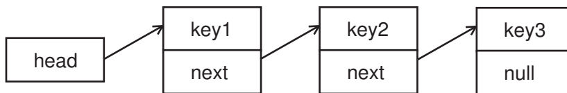
Рис. 2.3: Общий вид списка
