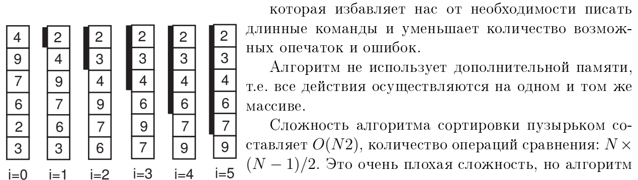
Рис. 4.2: Номер прохода. Отсортированная часть выделена полосой
