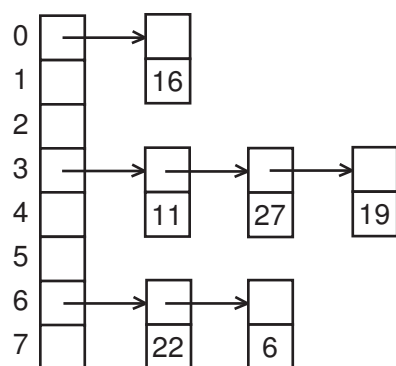
Рис. 2.6: Пример хеш-таблицы
