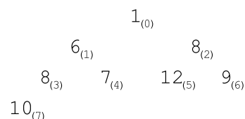
Рис. 2.1: Пример кучи
