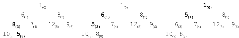
Рис. 2.2: Добавление в кучу (сравнимые элементы выделены)
